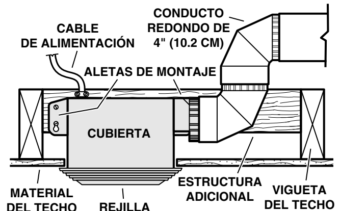
VIGUETAS DEL TECHO DE 24" (60.9 CM) Cubierta montada en otra estructura adicional
